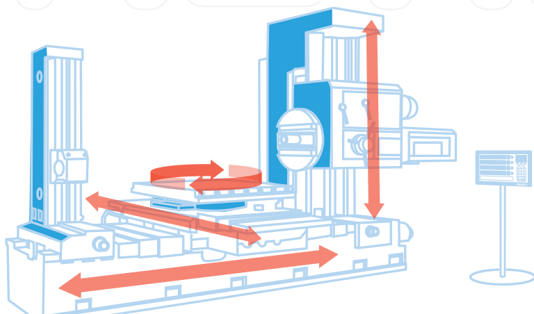
HORIZONTÁLNÍ VYVRTÁVAČKA
