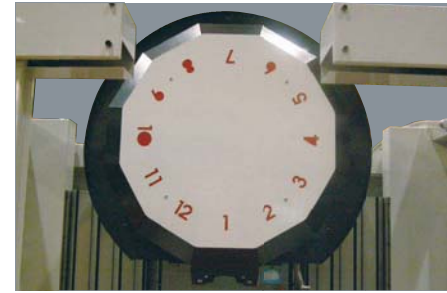
自動工具交換装置 12本 / 14本 (オプション) Automatic tool changer 12 tools / 14 tools (Option)
