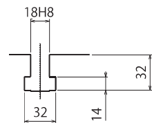
T溝寸法 / T slot
