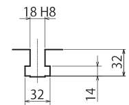
T溝寸法図 / T slot
