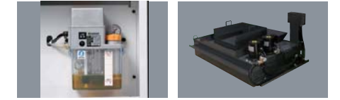
自動潤滑油装置 Automatic lubrication unit クーラントタンク Coolant tank
